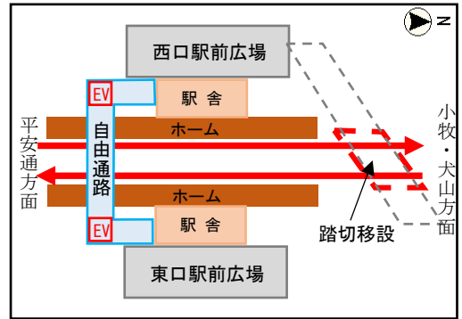
計画図（相対式ホーム・地上駅）
